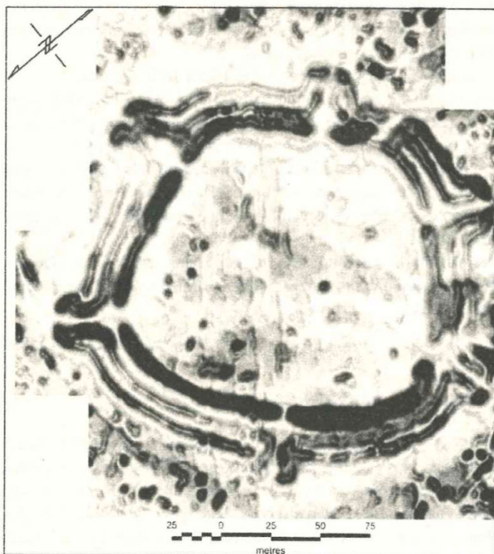
Obr. 1 Goliano. Mapa magnetických izolíní získaná nad neolitickým rondelom
